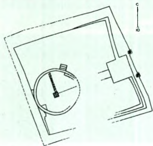
Уйбатский город. План храма Миропорядка (840–841)
